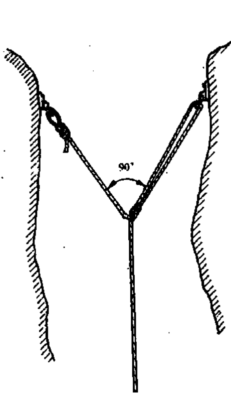
Фиг.25 Закрепване "У" между вертикални стени
