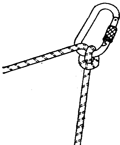
Фиг. 39. Спирачен възел
