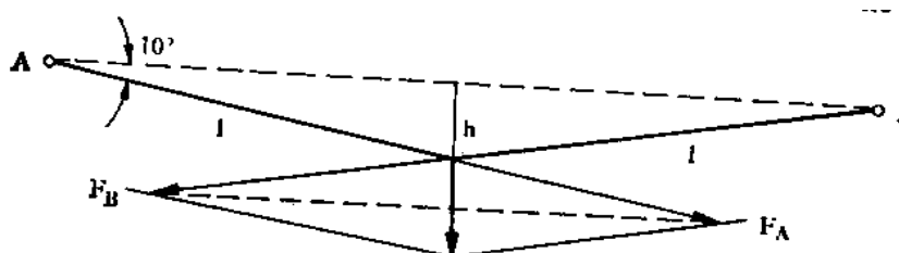
Фиг. 21. Схема за силите при натоварване на хоризонтално опънато въже
