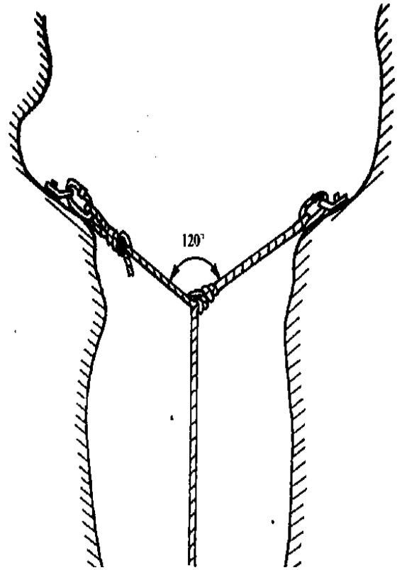
Фиг.25 Закрепване "У" между вертикални стени
