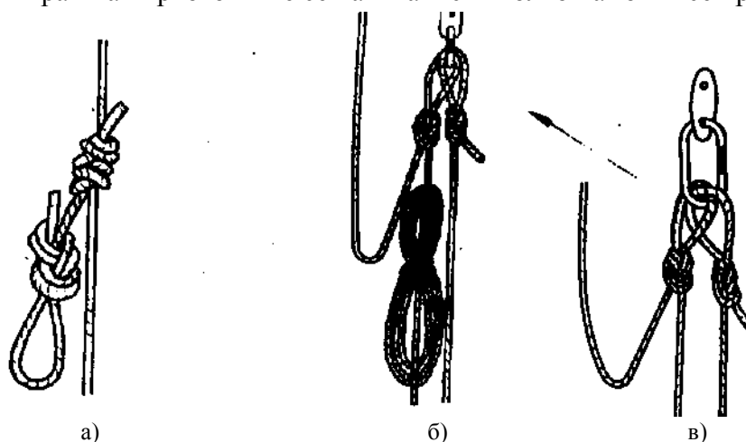
Фиг. 20. Свързване на две въжета: а) — камбана; б) и в) — към междинно закрепване
