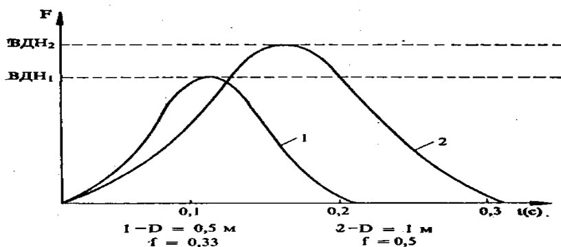
Фиг 31. Теоретични криви на ВДН при еднакви значения за С и F, но различна големина на «корема» D
