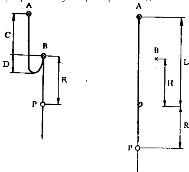
Фиг. 28 Фактор на падане при разрушаване на междинно закрепване
