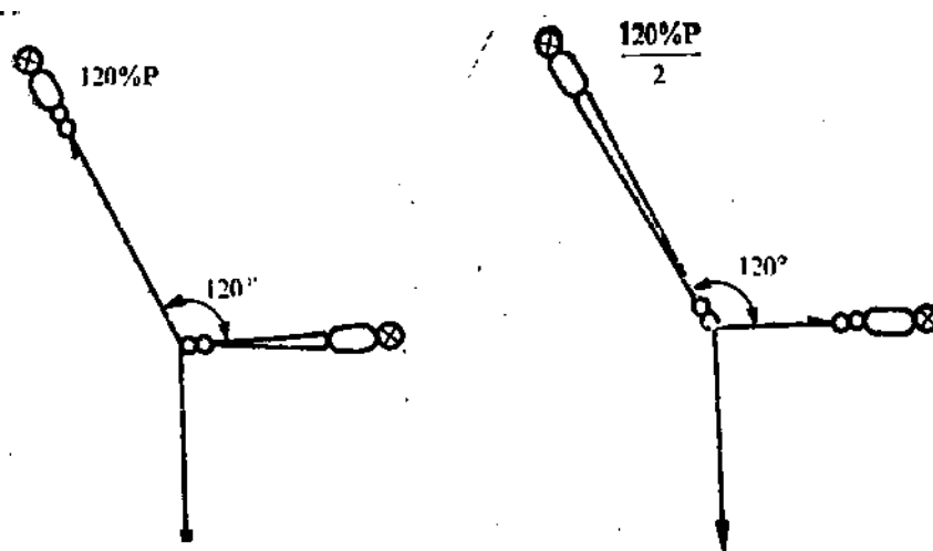
Фиг.23 Намалване на натоварването чрез вдвояване на въжето, фиксирано към по-висока опора на закрепването.
