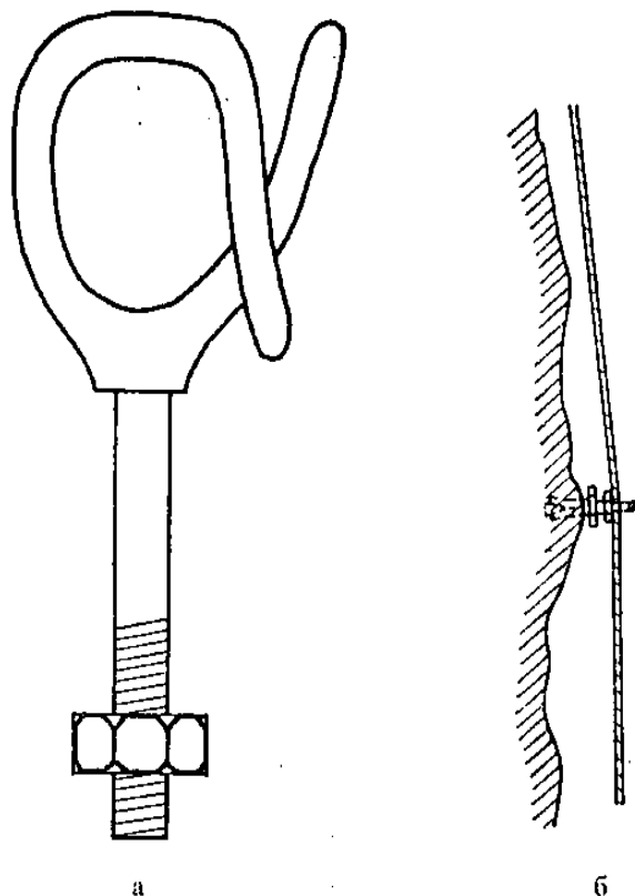
Фиг. 18 Отклонител а-общ вид; б-начин за използване
