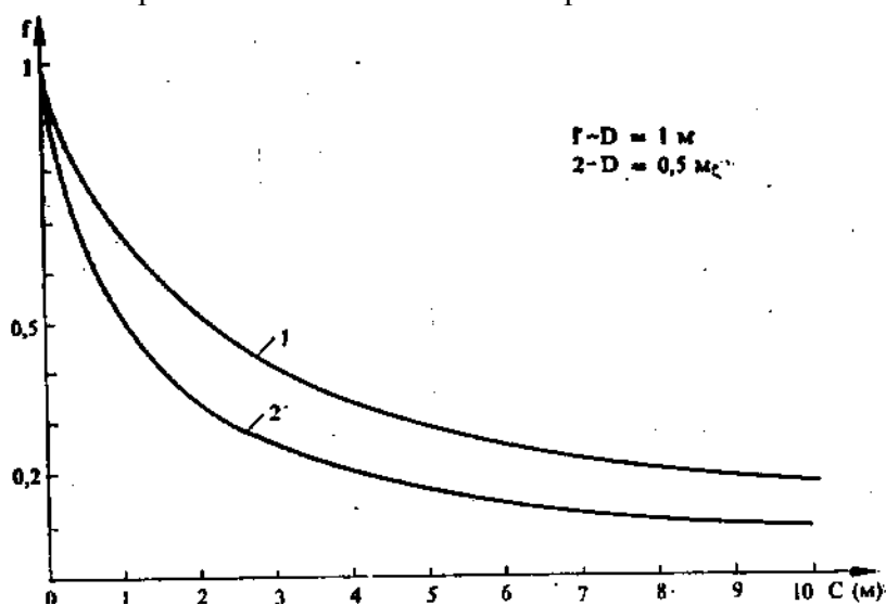
Фиг. 29. Зависимост на фактора на падане от дължината на въжето C над междинното закрепване и големината на «корема» D
