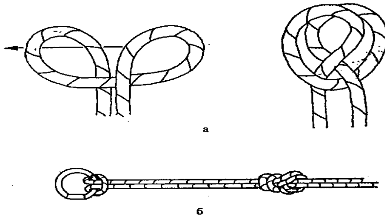
Фиг. 42. Помощни възли: а)- стреме; б)- котвена примка
