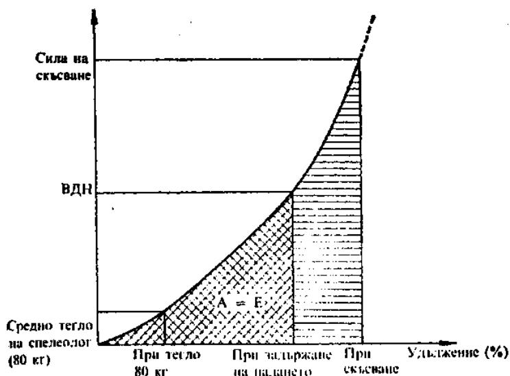
Фиг. 2. Удължение и работа на въжето при
